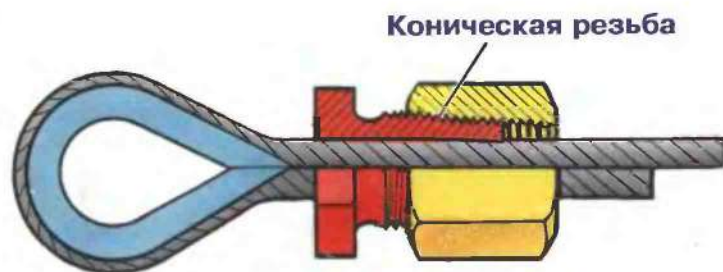
Цанговый захват
