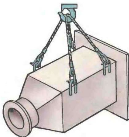
СТРОПОВКА ДЕТАЛИ СТАНКА ДВУМЯ ДВУХПЕТЛЕВЫМИ СТРОПАМИ
