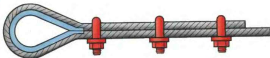
Винтовыми зажимами
