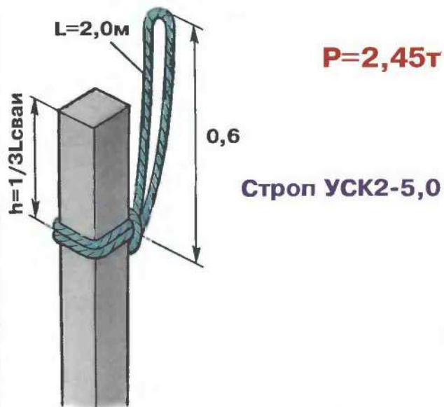
3. Железобетонная свая
