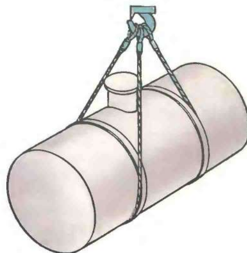
СТРОПОВКА ЦИЛИНДРИЧЕСКОГО РЕЗЕРВУАРА ДВУМЯ ДВУХПЕТЛЕВЫМИ СТРОПАМИ
