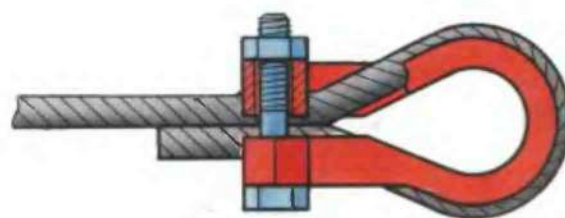
Коушный разъемный захват
