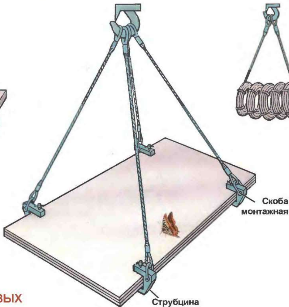
ПАКЕТ ЛИСТОВОЙ СТАЛИ
